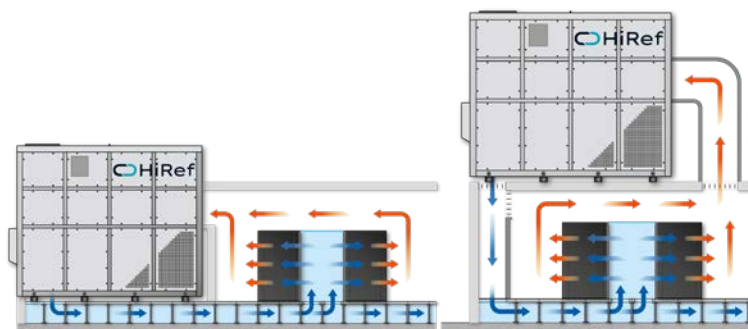
Esempio di utilizzo per Data Center di 1 MW (Ridondanza N+1) di Amsterdam @ 36°C - 25%; T aria in mandata 24°C; Max T aria in mandata 26°C
