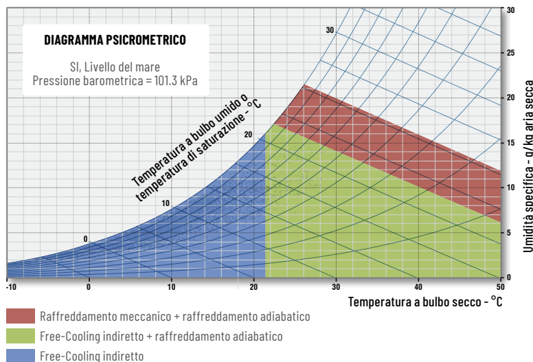
Esempio di utilizzo per Data Center di 1 MW (Ridondanza N+1) di Amsterdam @ 36°C - 25%; T aria in mandata 24°C; Max T aria in mandata 26°C
